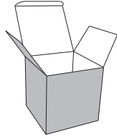
Die #336 18 pt 5" (w) x 5" (h) x 5" (d) Tuck closure
