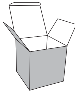
Die #336 18 pt 5" (w) x 5" (h) x 5" (d) Tuck closure
